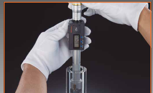
Typische Anwendung eines Holtests
