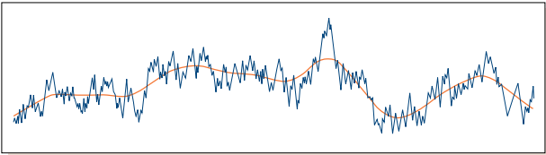
> Kuva 1: Primääriprofiili ja keskiarvo primääriprofiilin ( \lambda_c raja-arvo) suodattimelle
