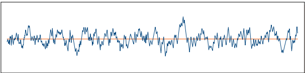
> Kuva 2: Karheusprofiili ja sen keskiarvo (primääriprofiilin ylipäästösuodatus raja-arvo-aallonpituudella \lambda_c )
