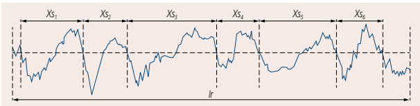
> Kuva 8: Keskimääräinen urien väli R_{Sm} on profiilielementtien välien X_{sj} keskiarvo
