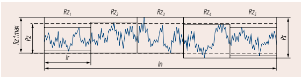
> Kuva 7: Karheusprofiilin kokonaiskorkeus R_t , karheuden keskimääräinen syvyys R_z ja karheuden maksimisyyvyys R_{z1max}
